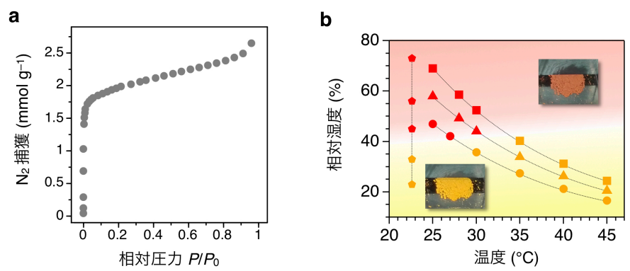
図 2 (a) -196\text{ }^{\circ}\text{C} における VPC-1 の窒素ガス吸着等温線。(b)多孔質結晶 VPC-1 の発色に関する相対湿度-温度相図。●、▲、■: 25\text{ }^{\circ}\text{C} における相対湿度 47, 58, 67%の状態から湿度を制御せずに温度を変化させたときの VPC-1 の色変化。五角形: 温度一定( 22.6\text{ }^{\circ}\text{C} )条件で相対湿度を変化させたときの VPC-1 の色変化。内挿写真は赤色および黄色の状態の VPC-1 粉末の写真。
