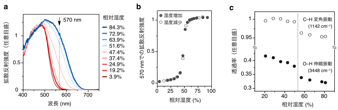
図 3 (a, b) VPC-1 粉末の拡散反射スペクトル(a)および波長 570\text{ nm} における拡散反射強度 (b) の湿度依存性。(c) VPC-1 粉末の FT-IR スペクトルにおける C-H 変角振動( \circ : 1142\text{ cm}^{-1} )および O-H 伸縮振動( \bullet : 3448\text{ cm}^{-1} )の湿度依存性。
