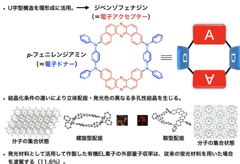
図1 今回開発した環状 TADF 材料の概略説明図
