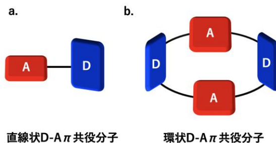
図2 TADF分子材料の構造
